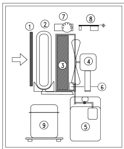
Fig. 1 Appareils avec flotteur d'arrêt
